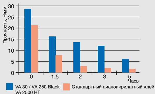
Кратковременное старение при +140 °C (+284 °F)
