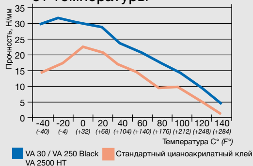
Прочность в зависимости от температуры
